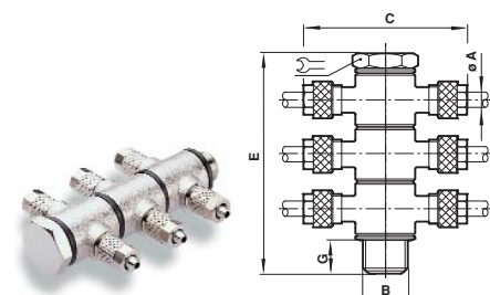
Banjo triplo a T
