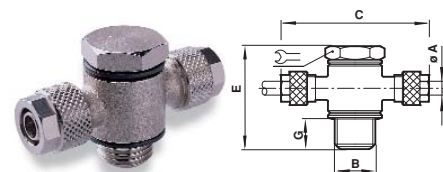
Assieme banjo a T
