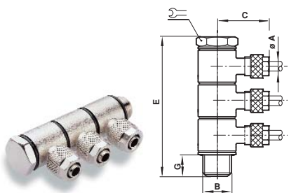
Assieme banjo a gomito triplo
